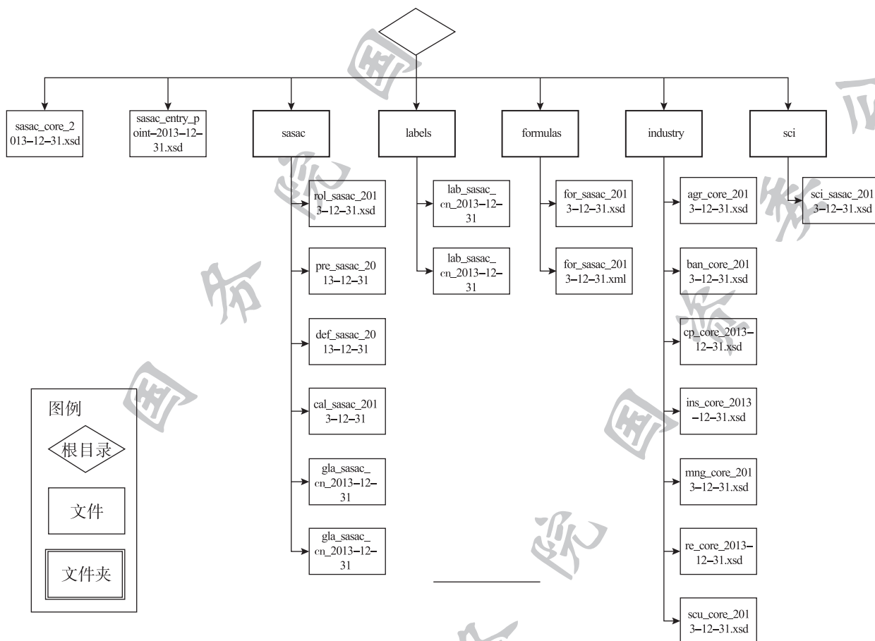
图 2 国资委扩展分类标准的文件夹和文件结构
