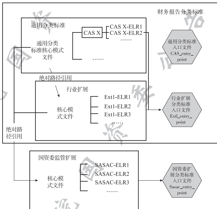
图 1 国资委扩展分类标准的设计架构
